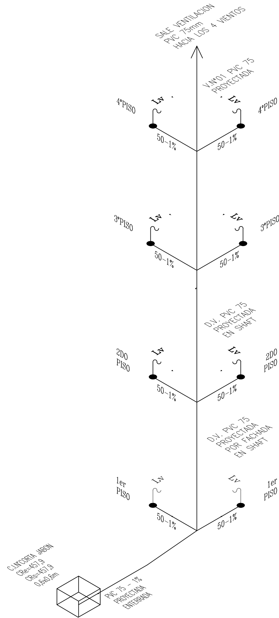
DETALLE PLANTA SISTEMA DE ALC, TRATAMIENTO AG Y RECIRCULACIÓN TRATAMIENTO | S/ESC
