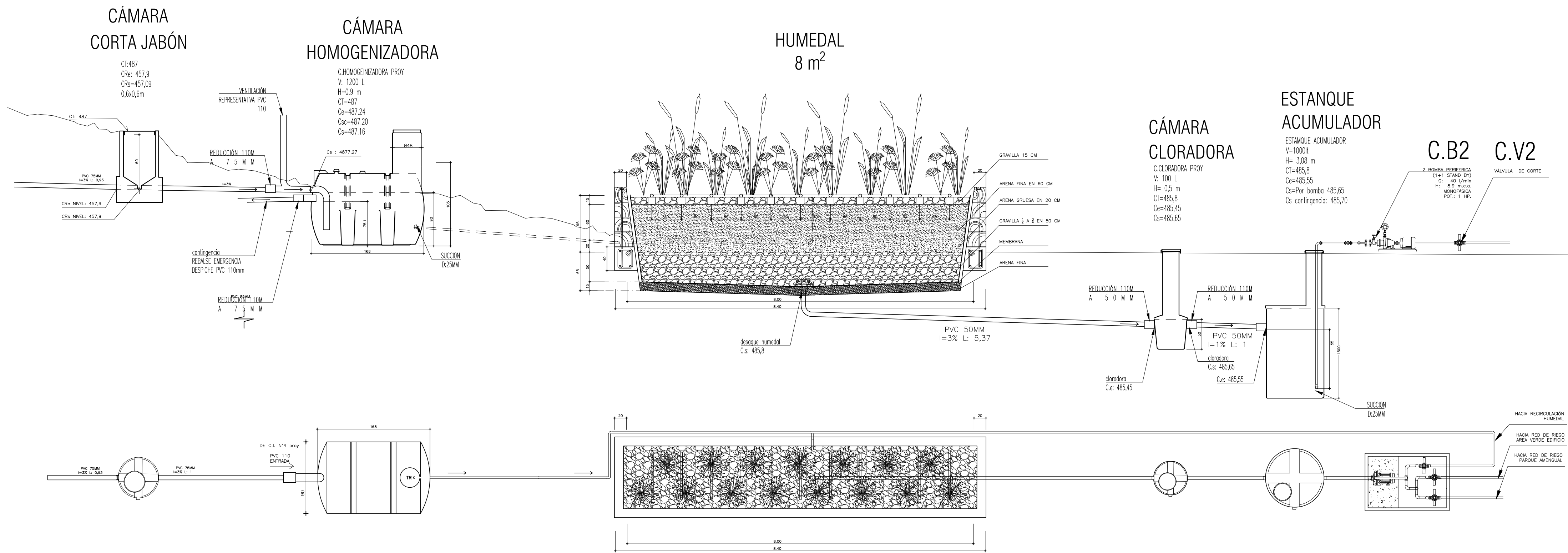
DETALLE ALZADO SISTEMA DE ALC, TRATAMIENTO AG Y RECIRCULACIÓN TRATAMIENTO | S/ESC
